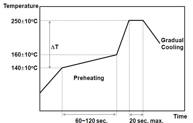
Vapor Reflow
