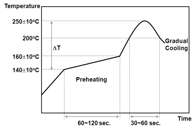
Vapor Reflow
